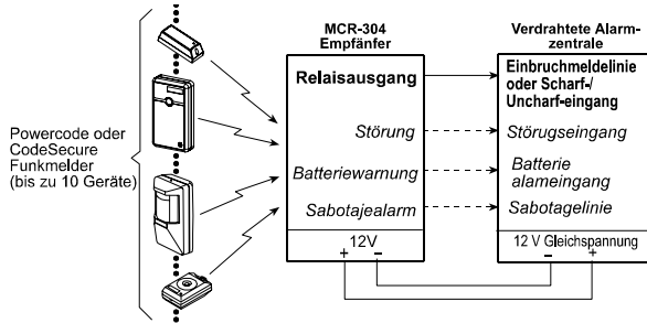
Abb. 1: Typische Anwendung des MCR-304
